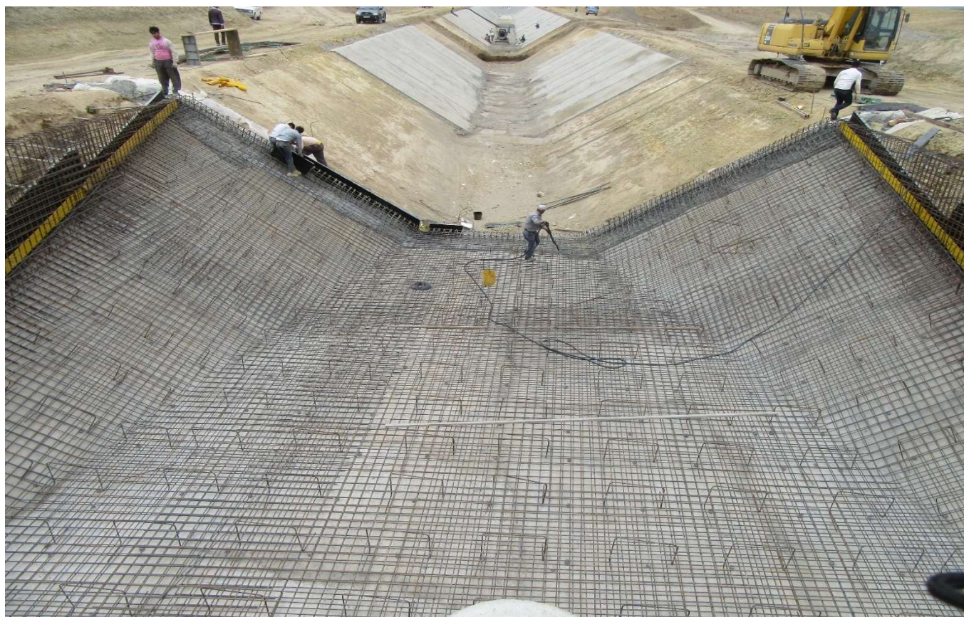
عملیات آرماتوربندی کف ترانزیشن ورودی سازه آمیل
