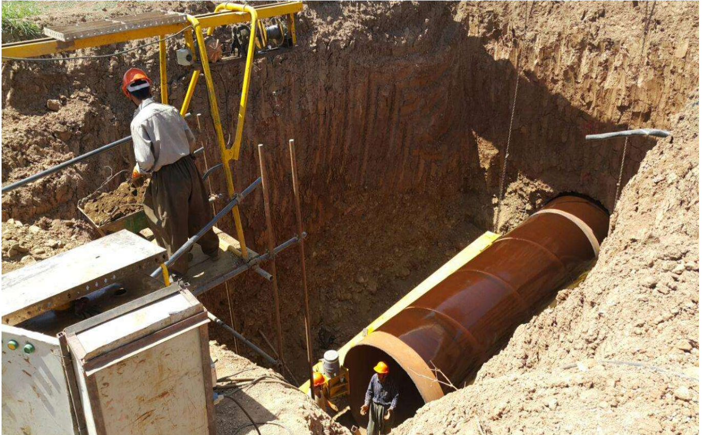
نمایی از اجرای عملیات لوله‌رانی با لوله فلزی به قطر ۲۰۰۰ میلی‌متر در تقاطع خطوط لوله و جاده پیرانشهر - سردشت
